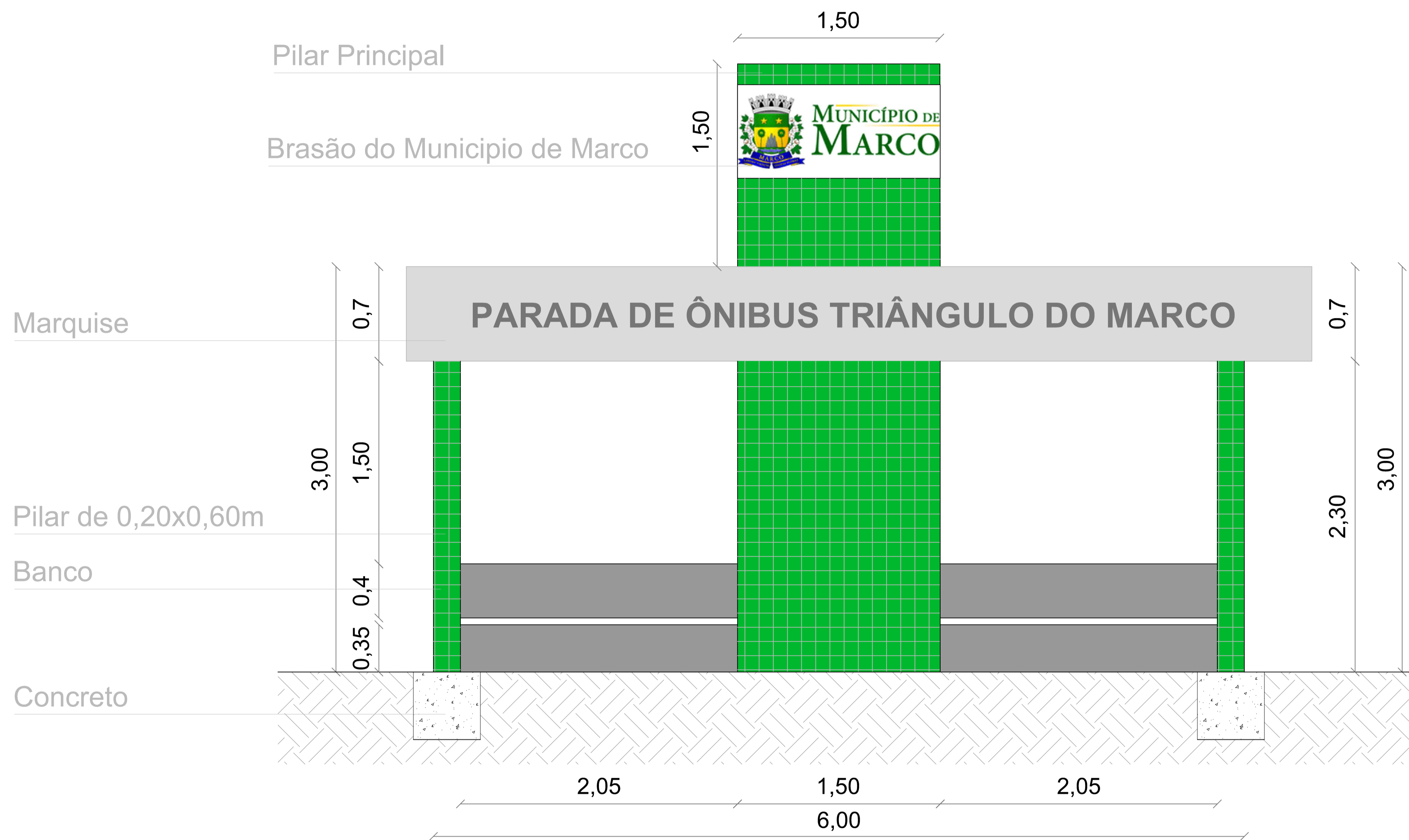
FACHADA / PARADA DE ÔNIBUS ESCALA 1/50
