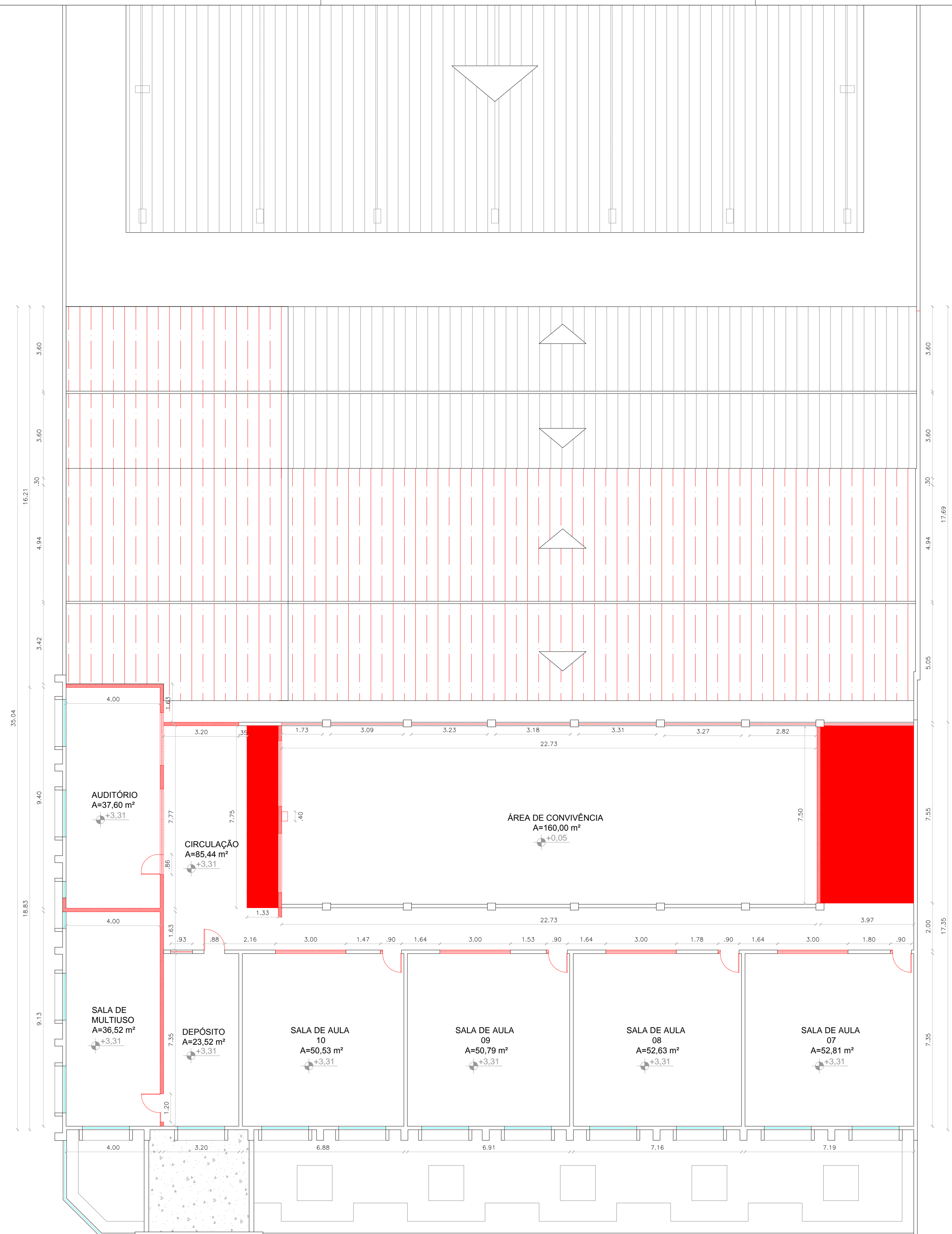
02 PLANTA DE DEMOLIÇÃO PAV. SUPERIOR Escala 1:100
