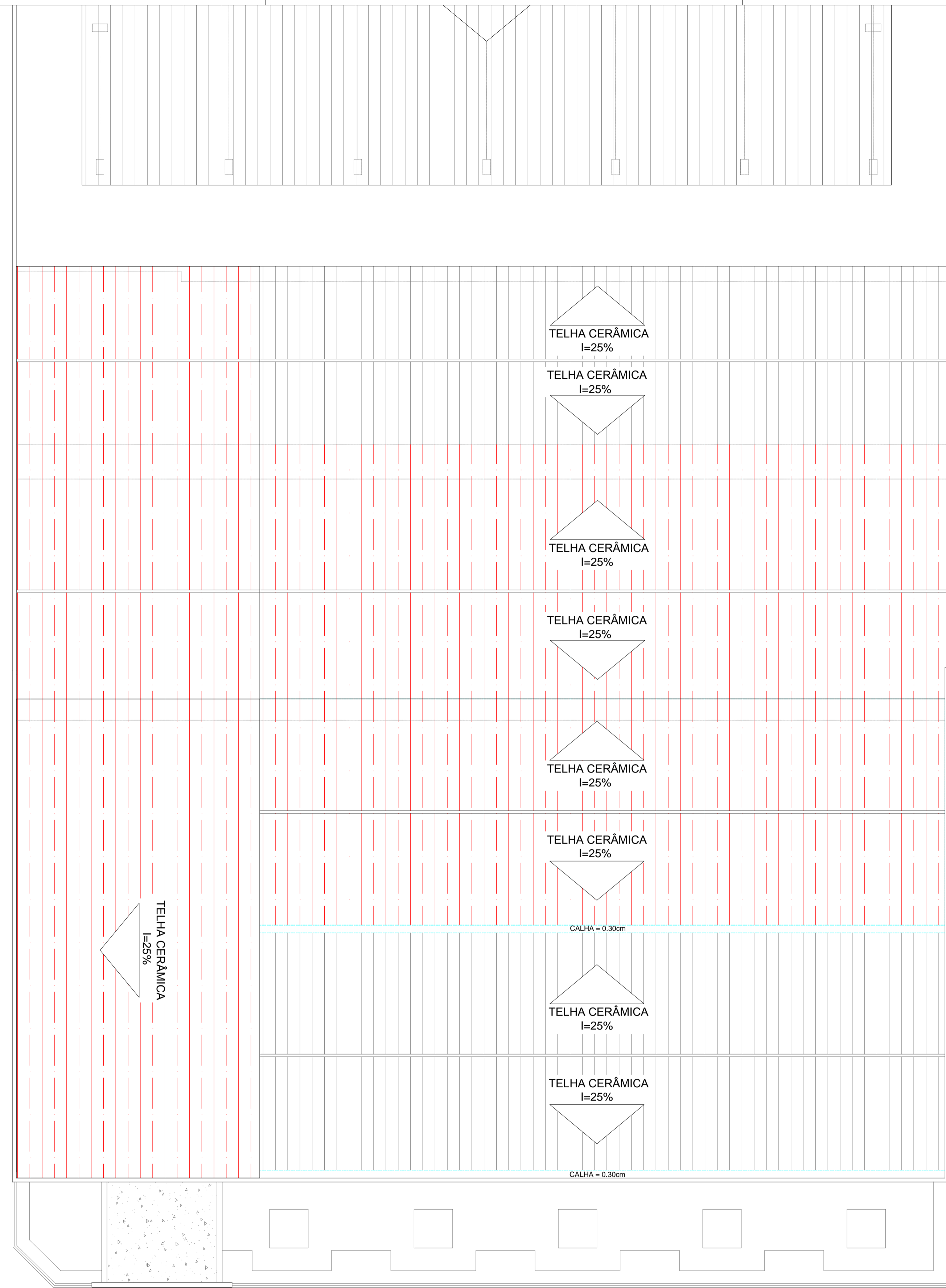
03 PLANTA DE DEMOLIÇÃO COBERTA Escala 1:100
