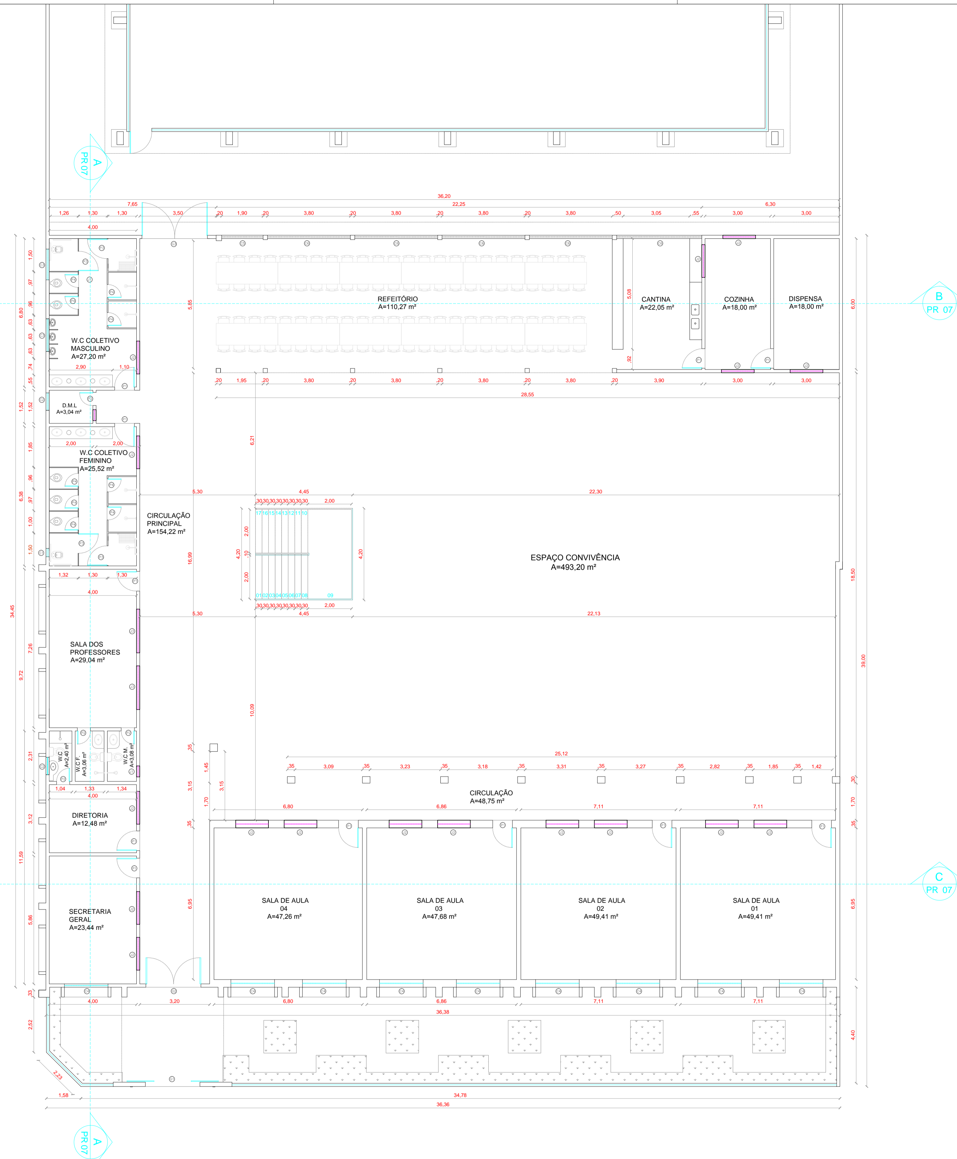
01 PLANTA BAIXA PAV. TÉRREO Escala 1:100
