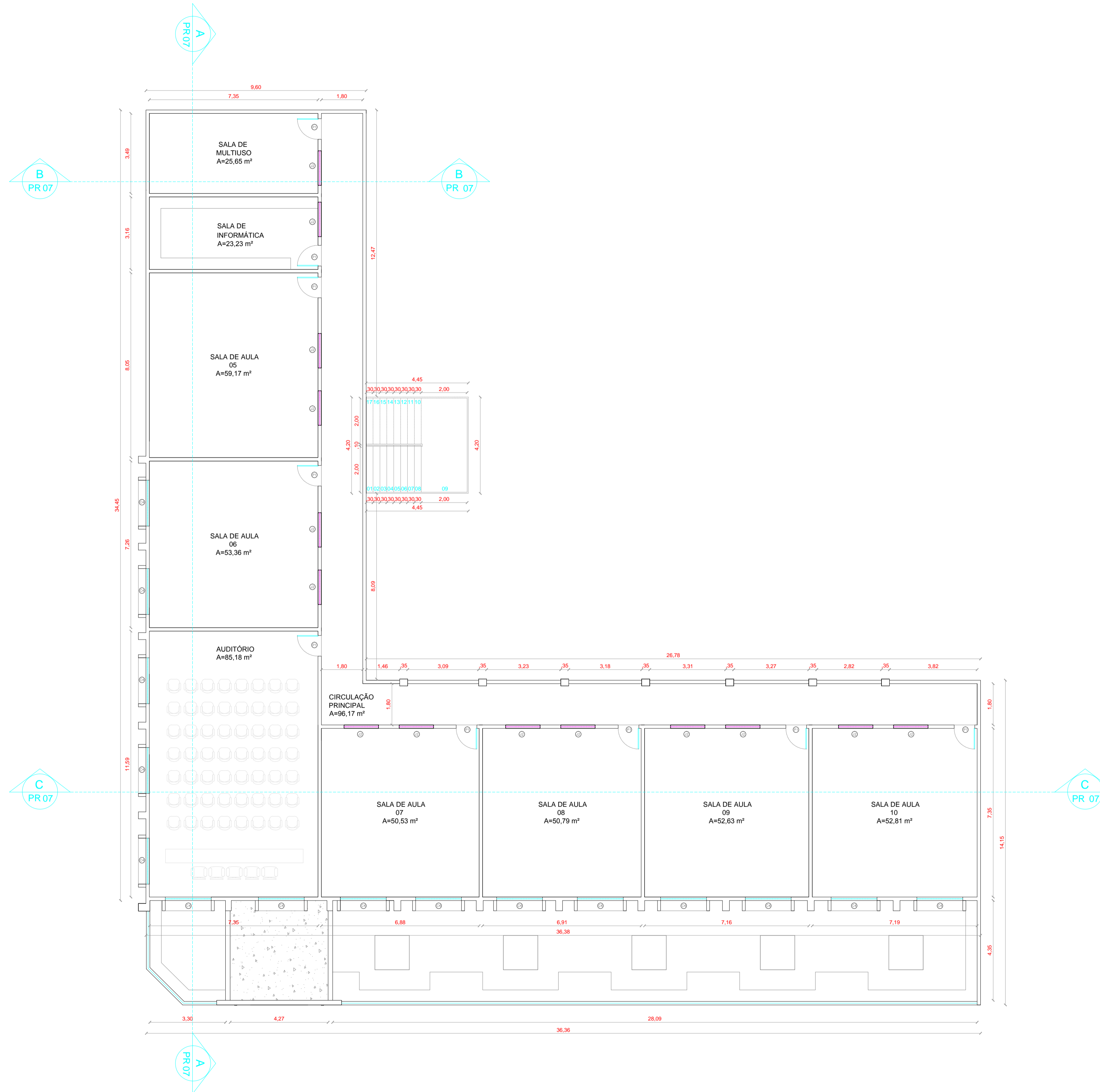
02 PLANTA BAIXA PAV. SUPERIOR Escala 1:100
