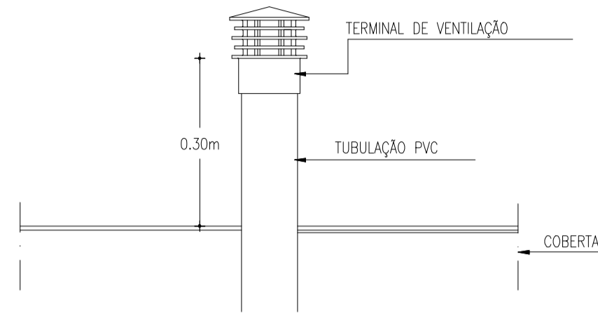
DET. TERMINAL DE VENTILAÇÃO ESCALA : S/E
