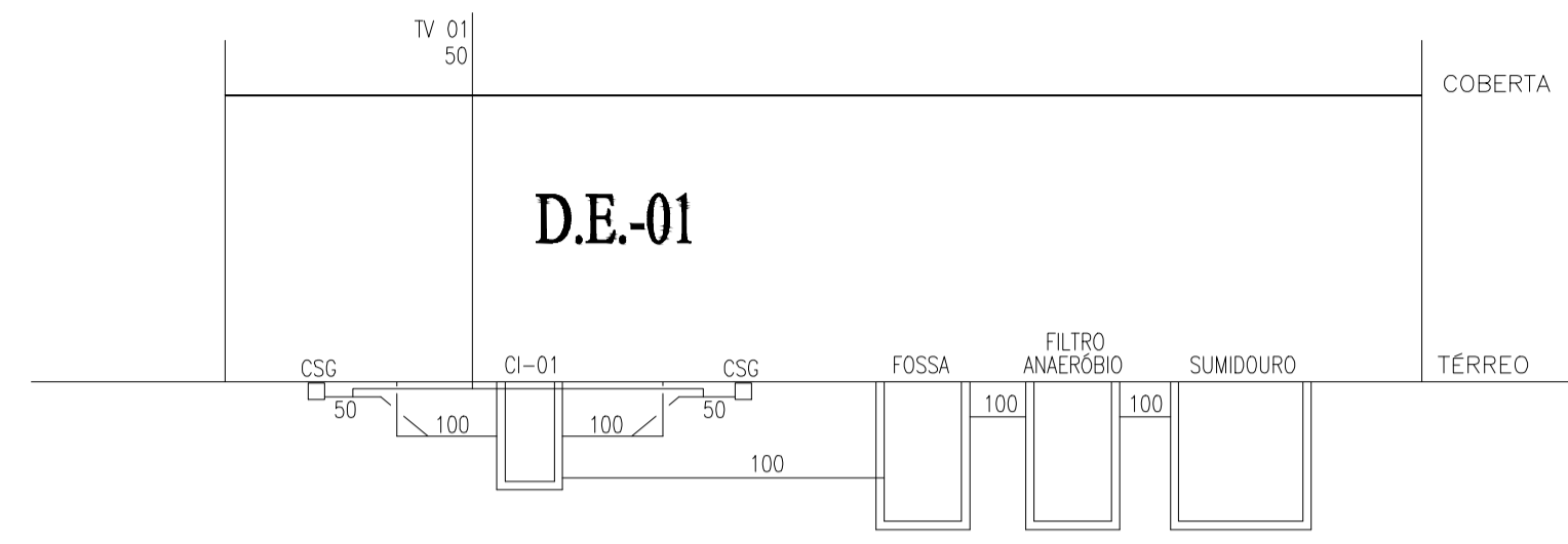
ESQUEMA VERTICAL DE ESGOTO ESCALA : S/E
