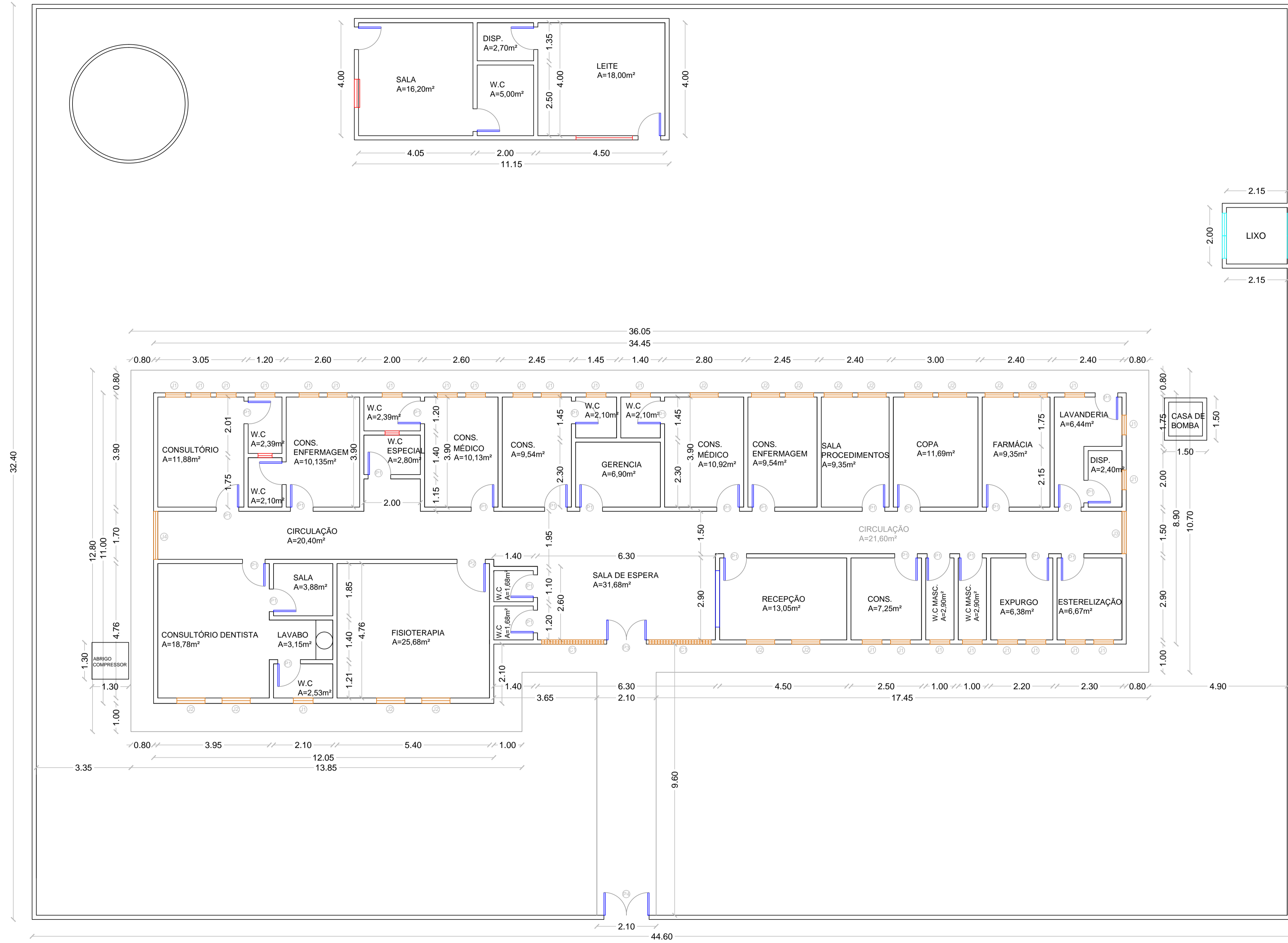
01 PLANTA BAIXA ESCALA 1:75
