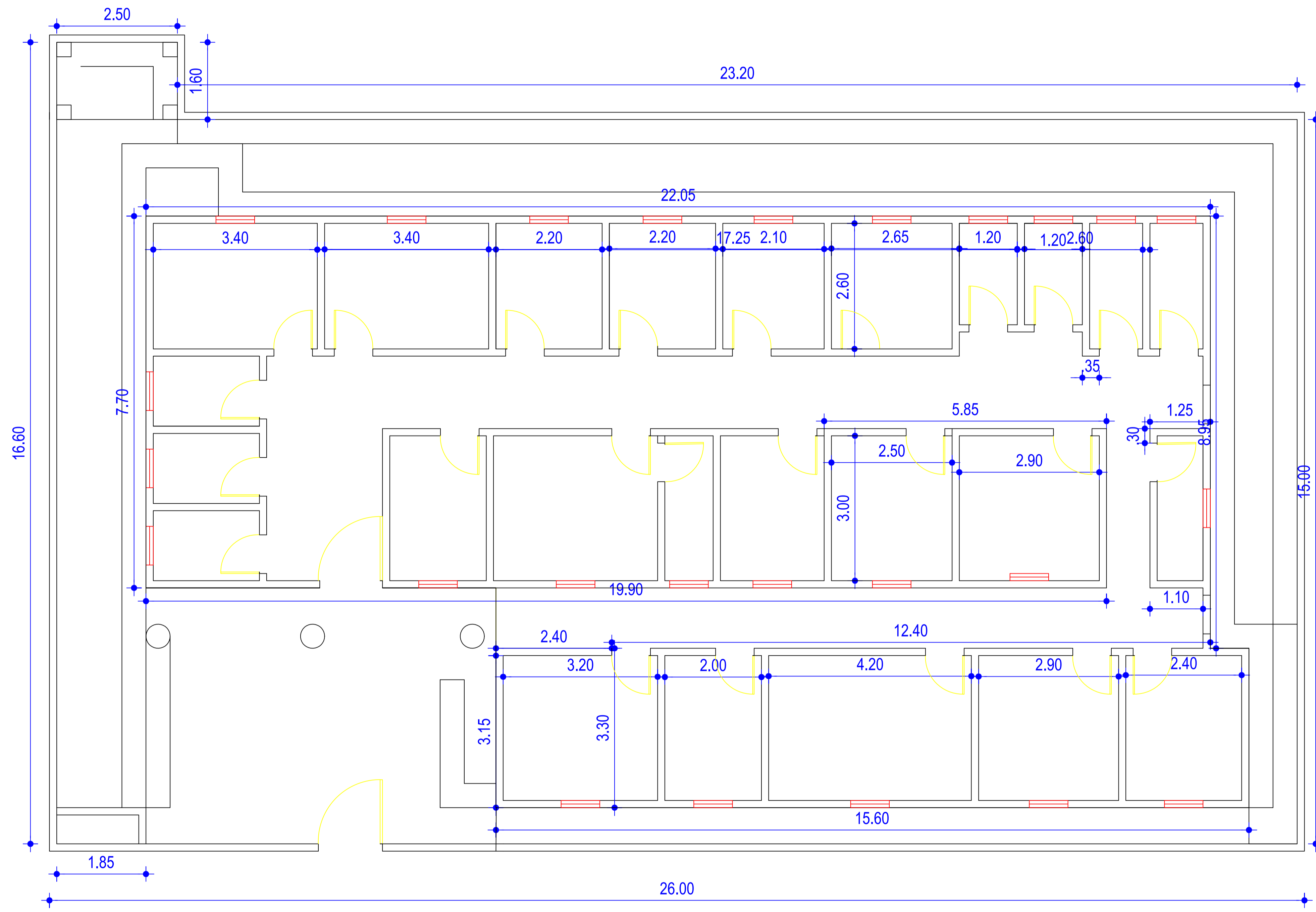
01 PLANTA BAIXA ESCALA 1:50
