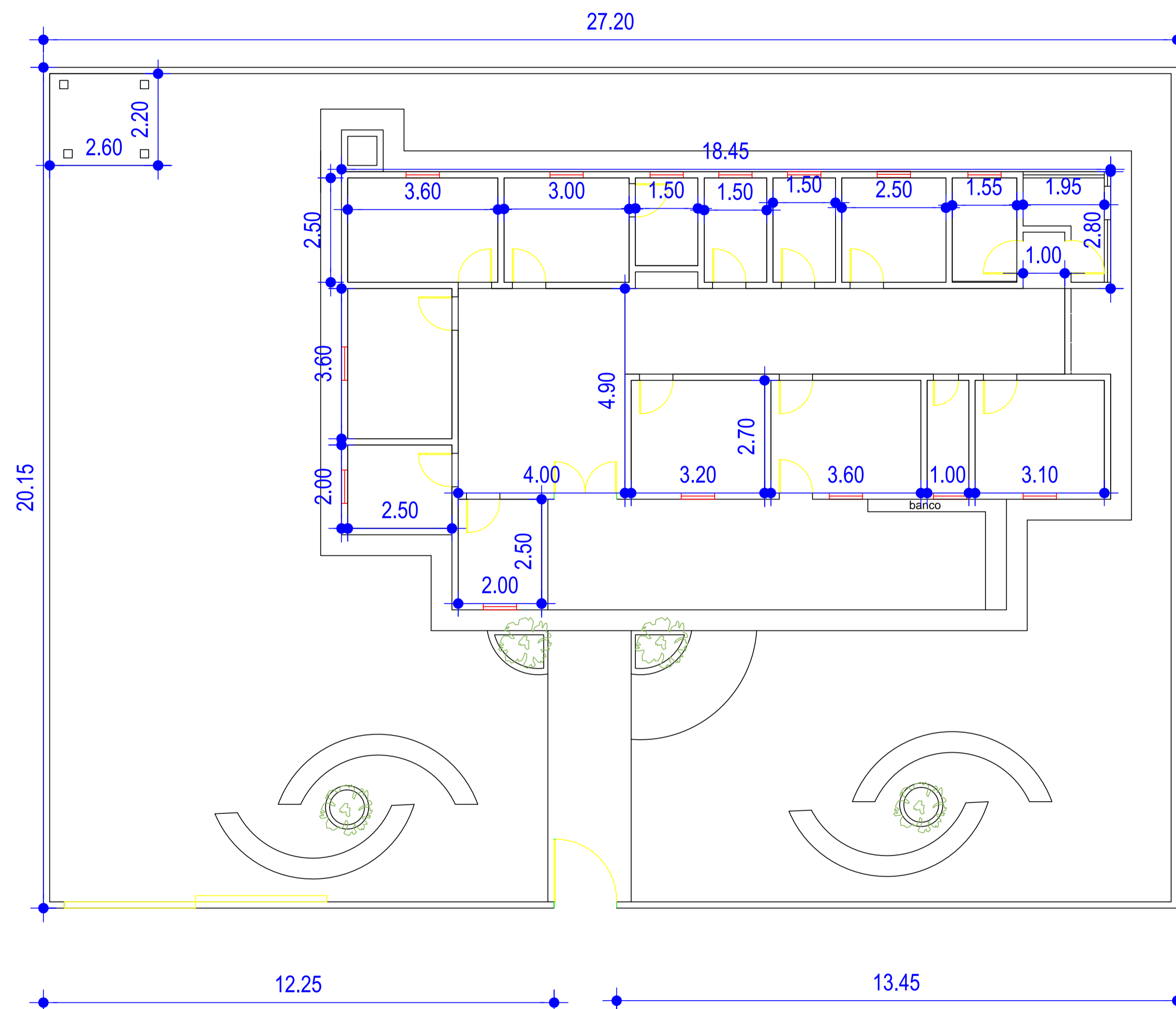
01 PLANTA BAIXA ESCALA 1:75
