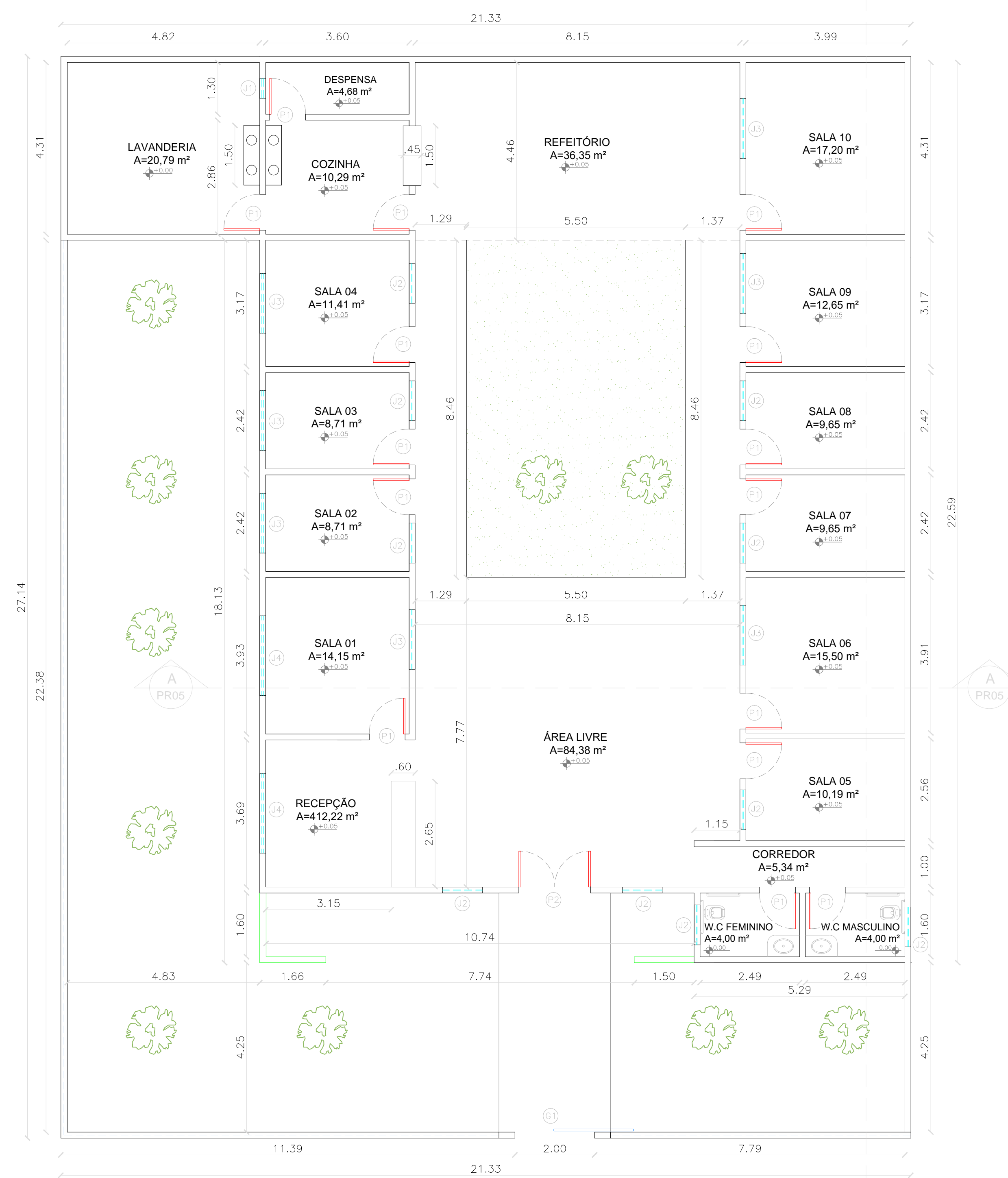
01 PLANTA BAIXA Escala 1:75
