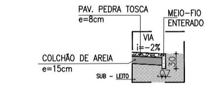
05 DET. MEIO FIO esc.: 1 / 75
