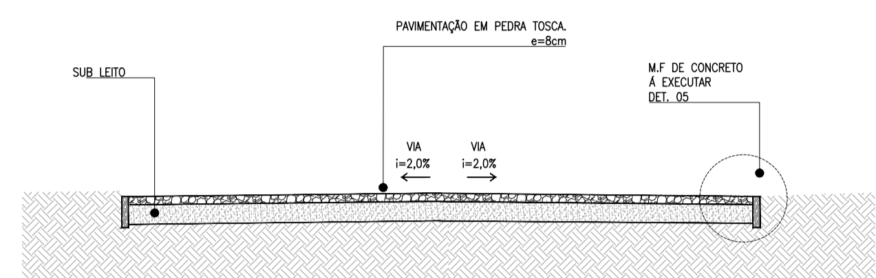
03 SEÇÃO TIPO 6m esc.: 1 / 50 • TRECHO 01: 0+0,00 - 8+0,00 • TRECHO 02: 532+3,00 - 540+3,00
