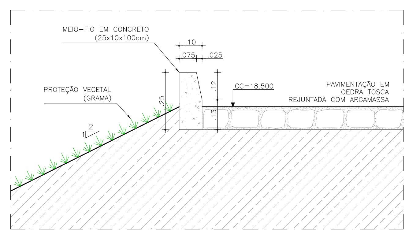
3 DETALHE: MEIO-FIO ESCALA: 1/10
