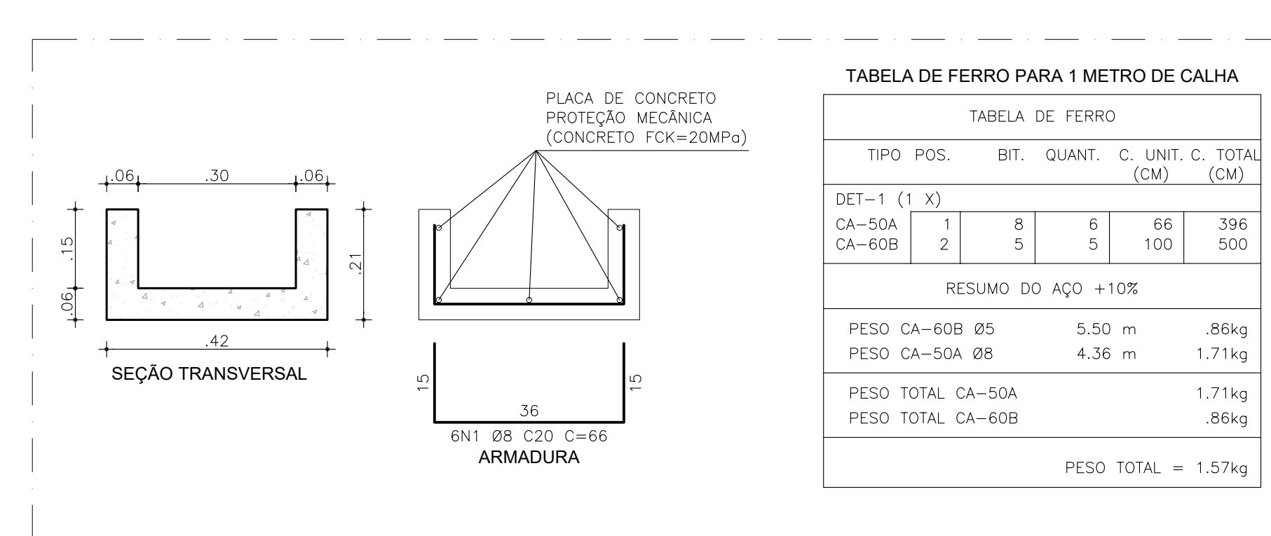
5 CANALETA: ESTRUTURAL ESCALA: 1/10
