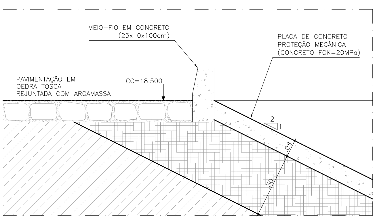
4 DETALHE: PLACA DE PROTEÇÃO ESCALA: 1/10
