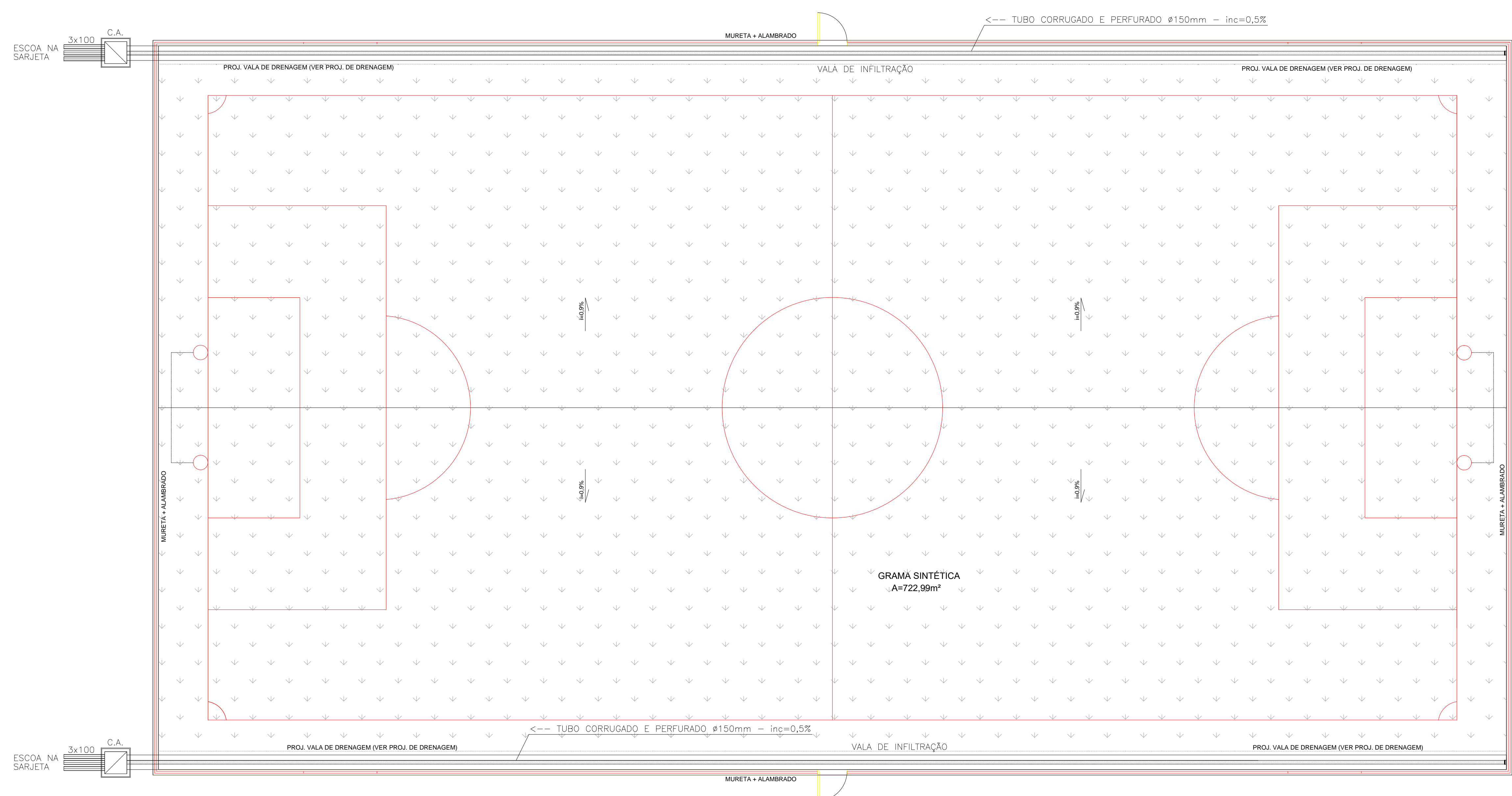
DRENAGEM ESCALA: 1/75
