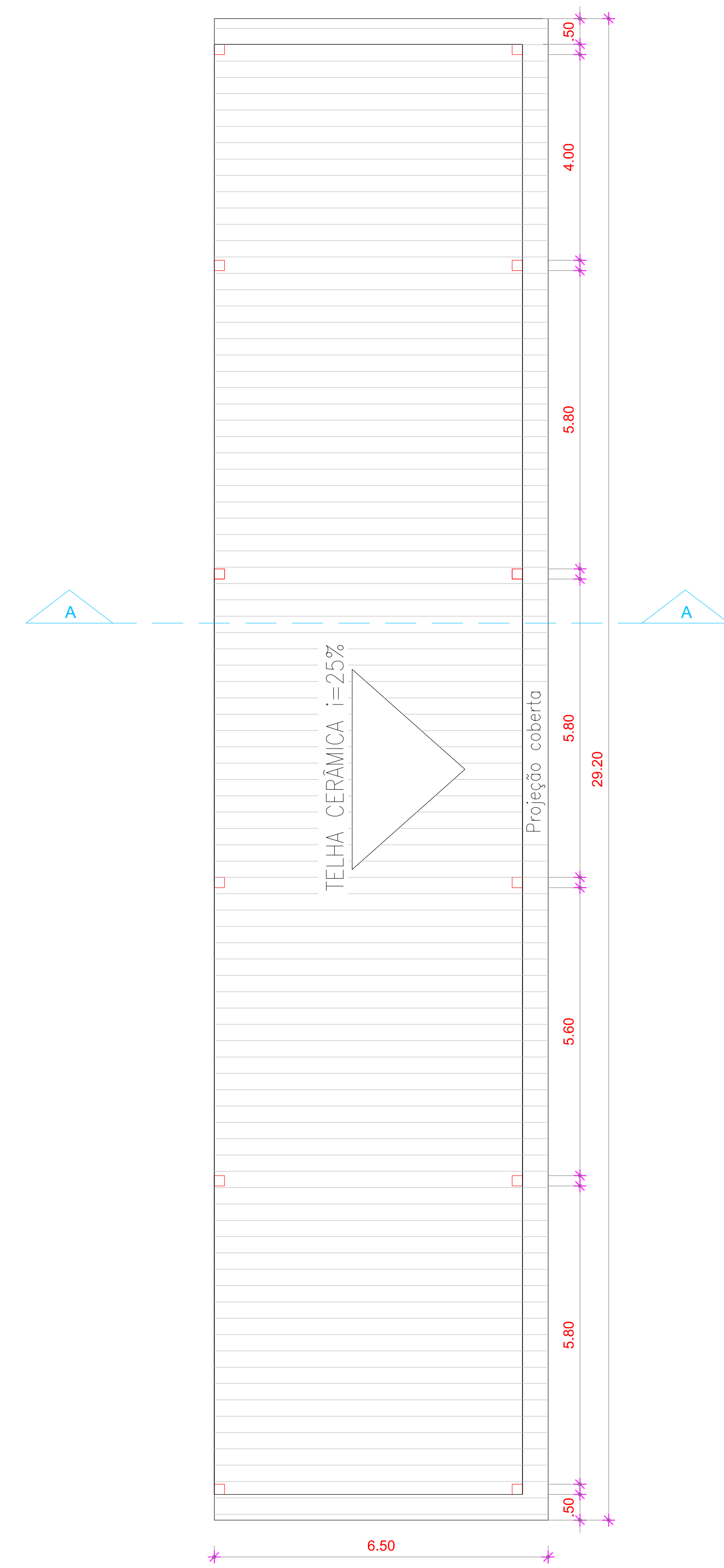
02 COBERTA 02 ESCALA: 1/100
