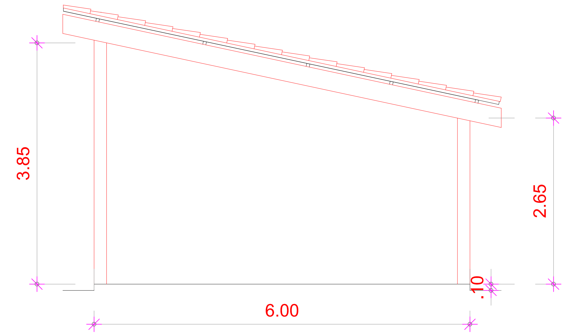
A CORTE-COBERTA ESCALA: 1/100
