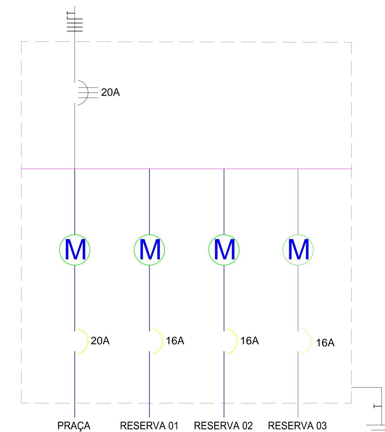
ESQUEMA UNIFILAR
