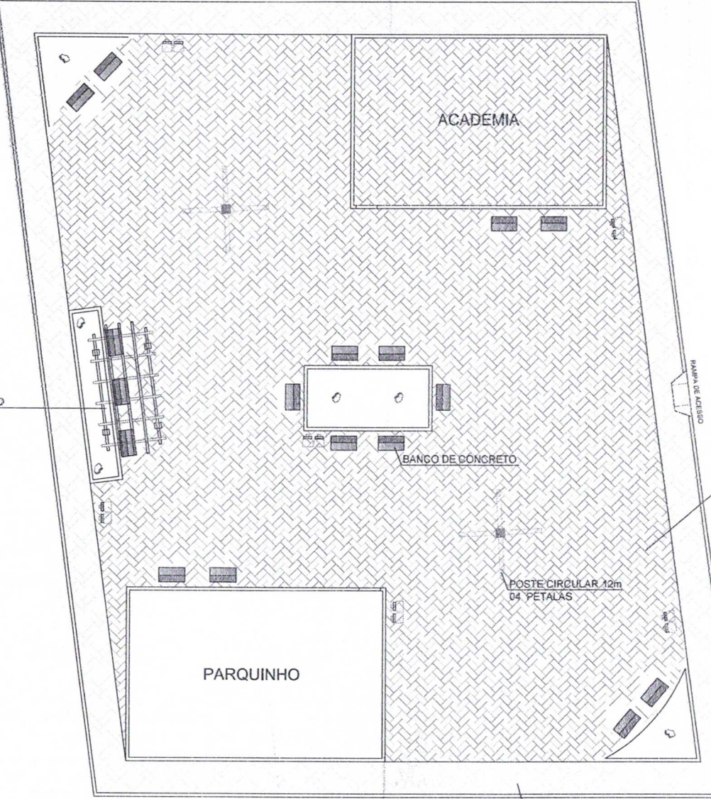
01 PLANTA LAYOUT ESCALA 1/100
