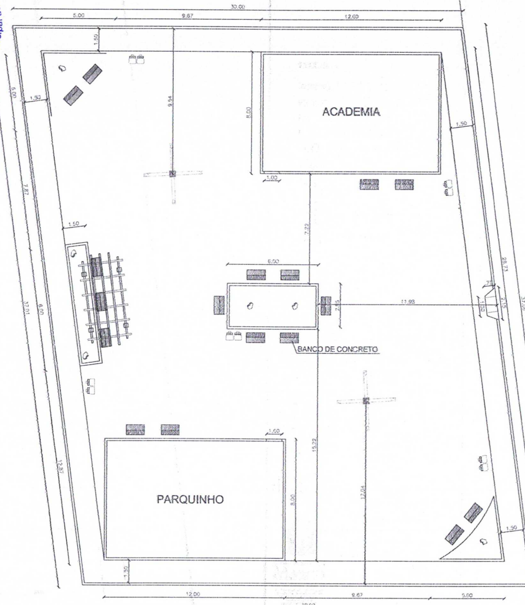
02 PLANTA COTADA ESCALA 1/100
