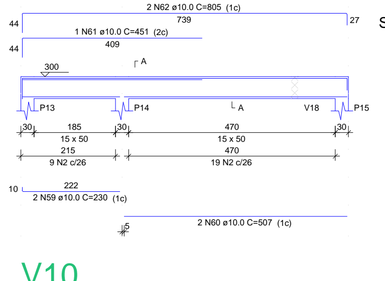
V10 ESC 1:100
