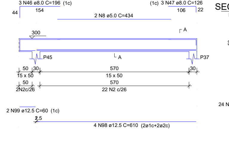
V25 ESC 1:100
