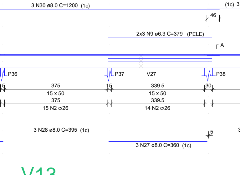
V13 ESC 1:100
