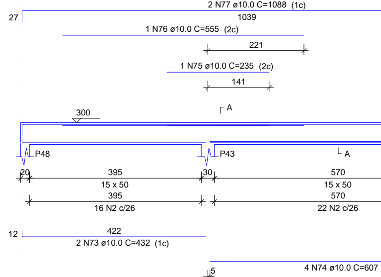
V27 ESC 1:100
