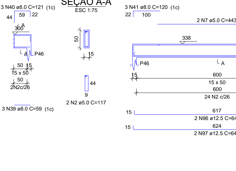
V28 ESC 1:100
