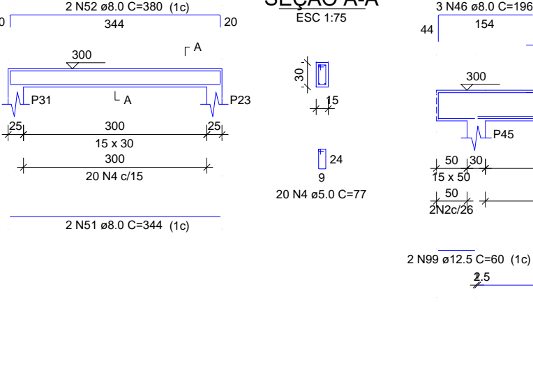
V24 ESC 1:100
