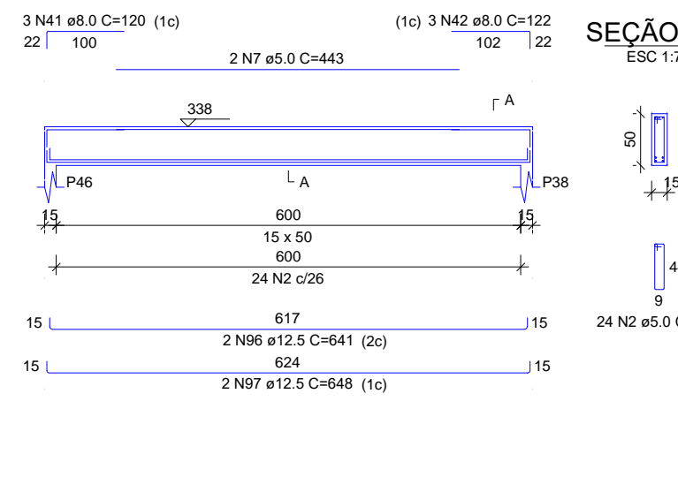
V29 ESC 1:100
