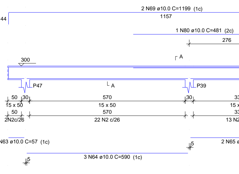
V30 ESC 1:100
