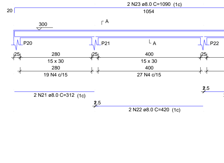
V7 ESC 1:100
