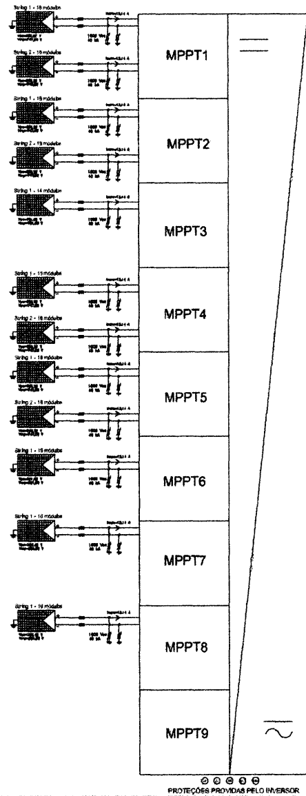
MÓDULO CANADIAN SOLAR - CS6W-545MS
