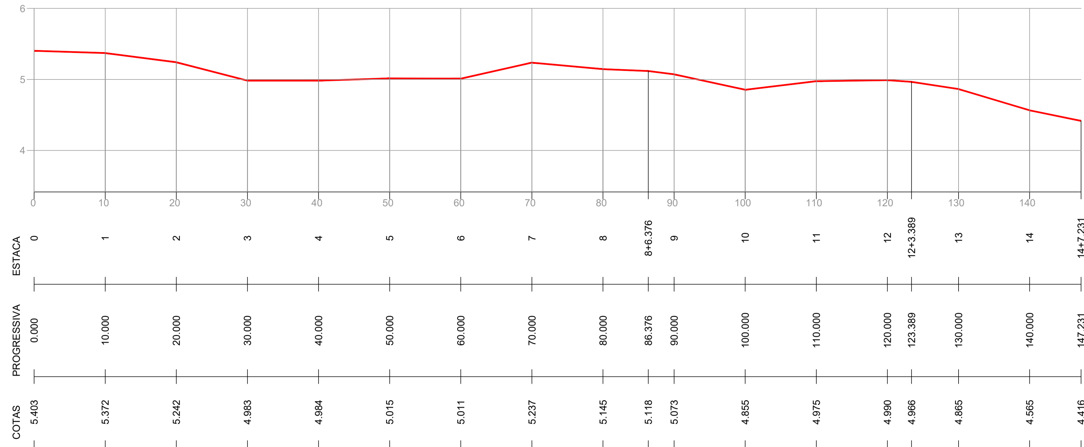
PERFIL LONGITUDINAL - RUA DA CAGECE
